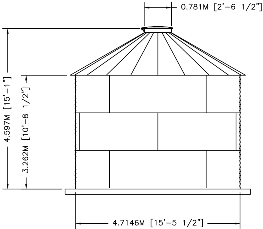
ELEVATION
